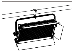
灯钩吊挂图
